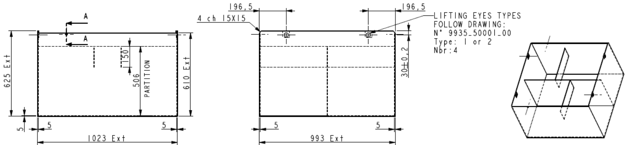
Afbeelding: Een schematische tekening van een speciale container op maat.
